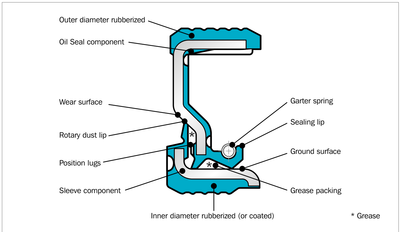
Figure 59: APJ Seal
